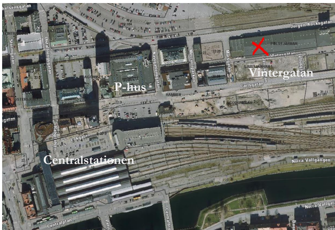
Översiktsarta Vintergatan
