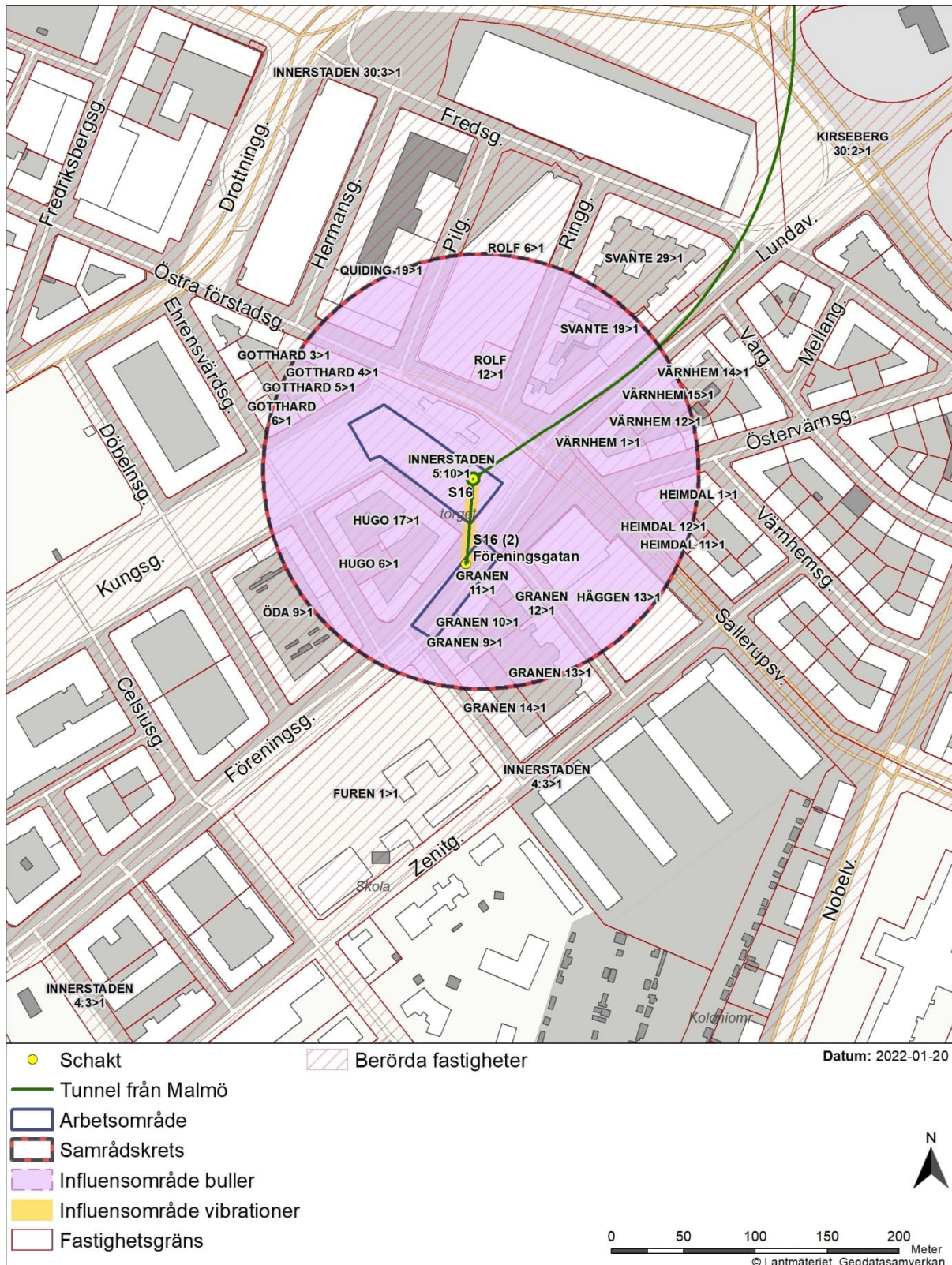
Figur 1 Arbetsområden samt påverkansområden för buller och vibrationer under byggskedet.
