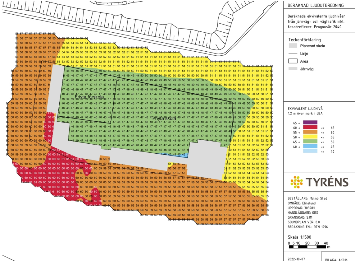
Bullerkarta som visar bullervärden för skolan och förskolas fastighet. Enligt bullerutredningen är skolan och förskolan inte beroende av annan utbyggnad för att klara riktvärdena för buller på friyta.
