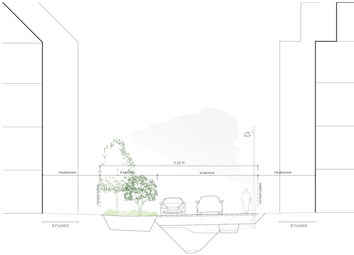
Ovan och under, två typsektioner för 11,0 meter breda lokalgator. Sektionerna visar att både trädplantering och ledningar och att gatorna kan vara med eller utan trottoarer.
