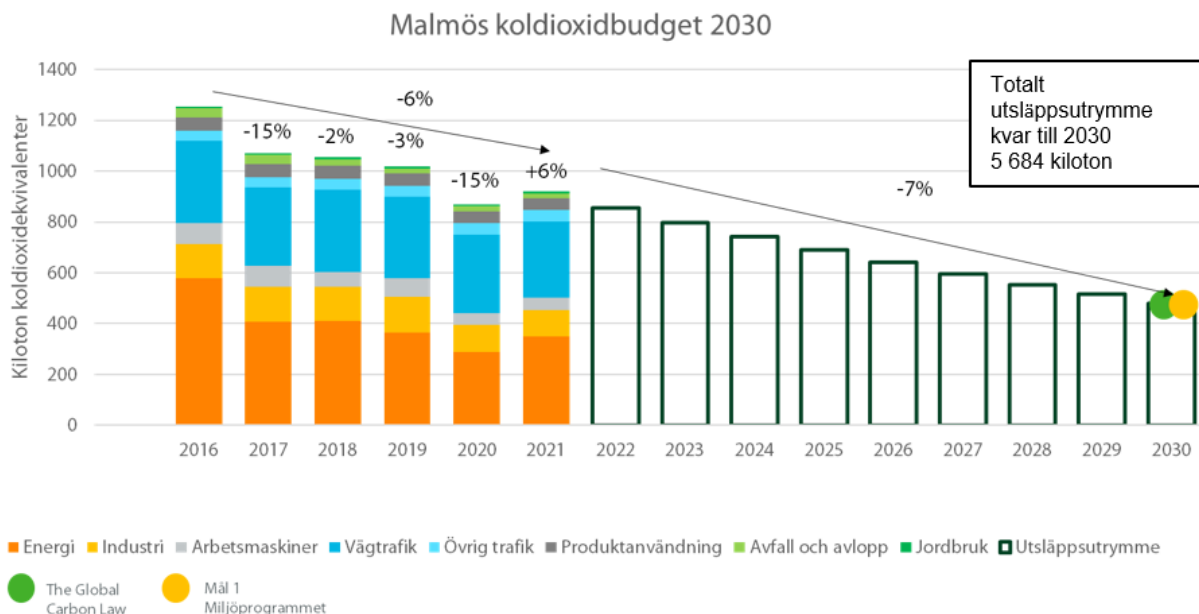
Figur 2. Malmös koldioxidbudget för de territoriella växthusgasutsläppen till 2030.
