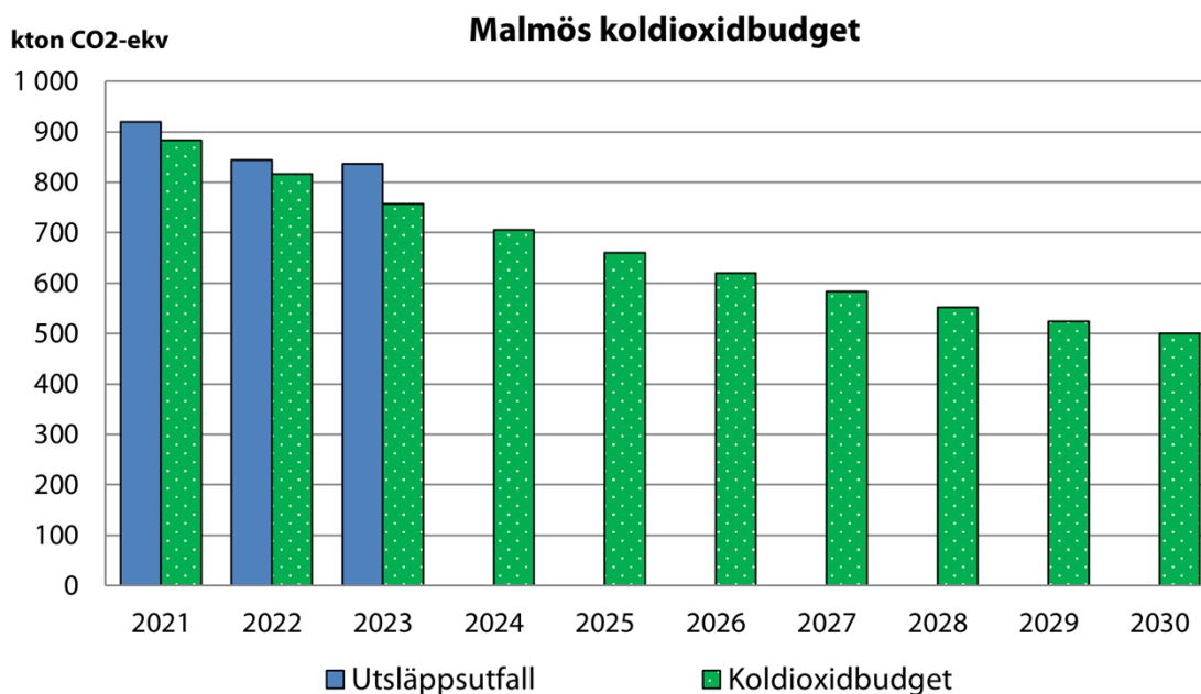
Diagram 2. Utsläpp av växthusgaser jämfört med Malmö koldioxidbudget 2021-2030.
