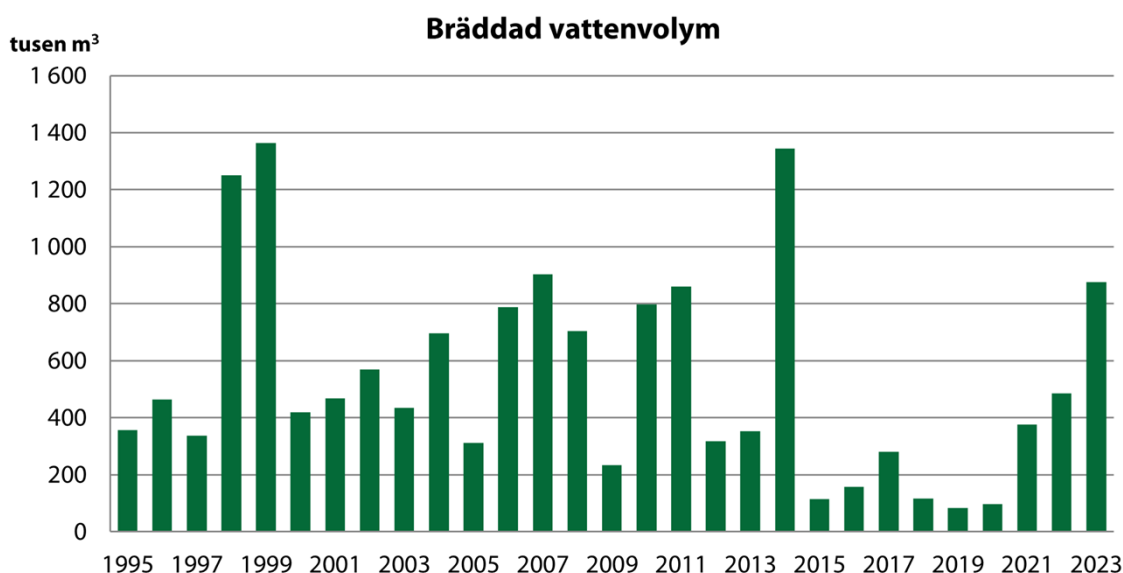
Diagram 11. Volym (m 3 ) bräddat vatten i ledningsnät och på avloppsreningsverk. Sammanställning av mängden vatten som bräddar vid reningsverk och på ledningsnät vilket redovisas i avloppsreningsverkens miljörapporter. Datakälla: VA SYD.
