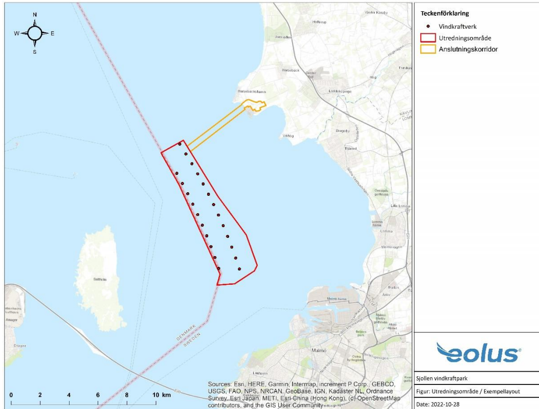
Figur 1: Översiktsskarta med utredningsområde, exempellayout med 23 vindkraftverk och anslutningskorridor till land.
