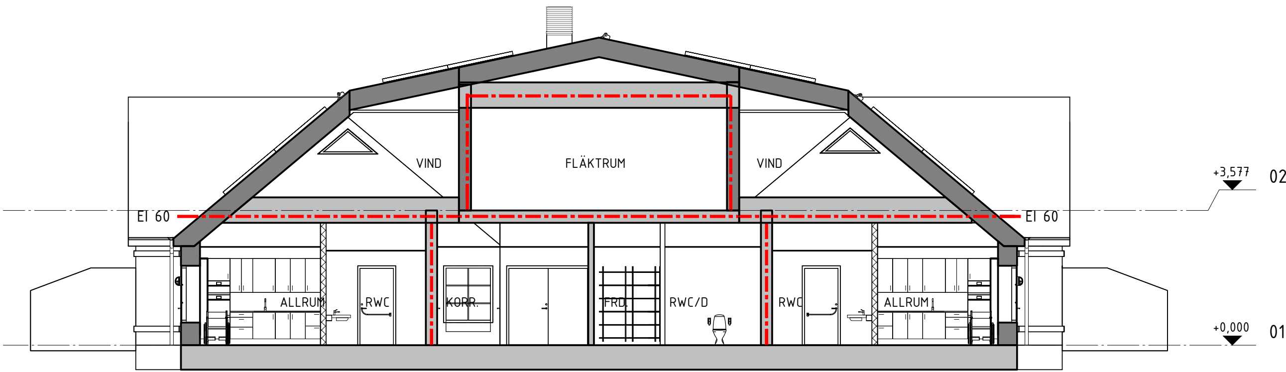
SEKTION C-C
