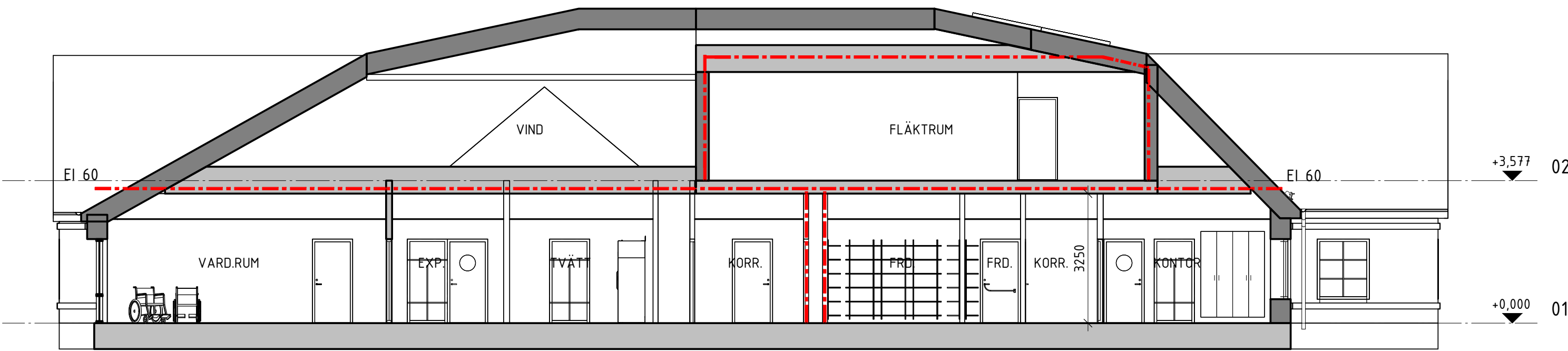
SEKTION A-A
