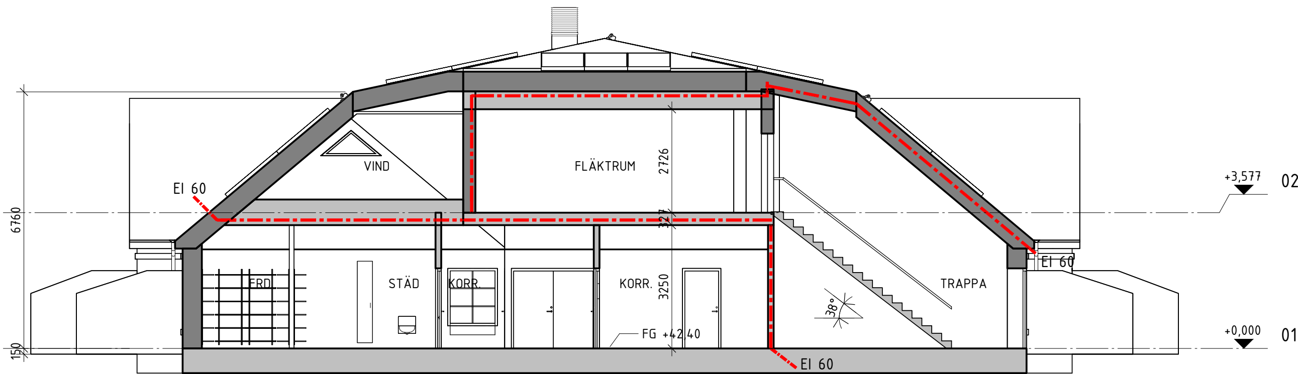
SEKTION B-B
