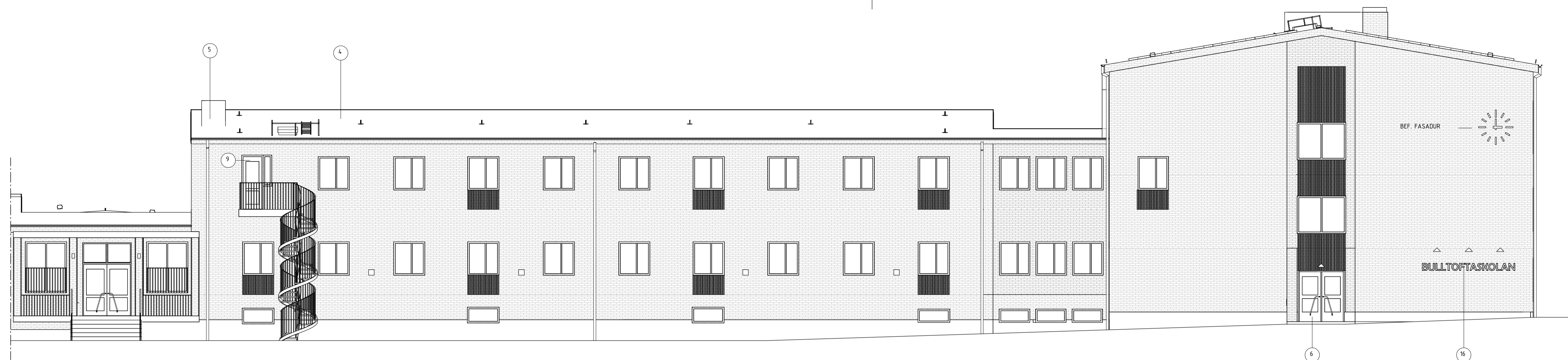
FASAD MOT NORR
