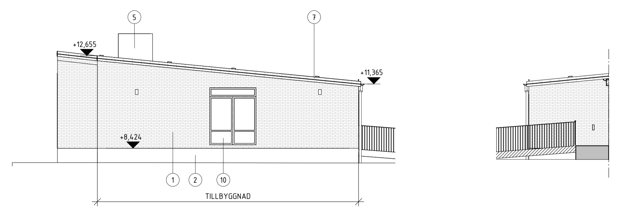
FASAD MOT ÖSTER
