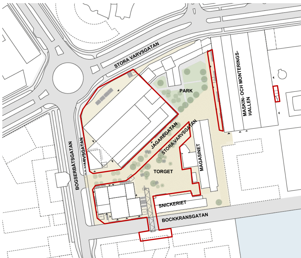
Strukturskiss för del av Varvsstaden med planområden markerat med röd linje.
